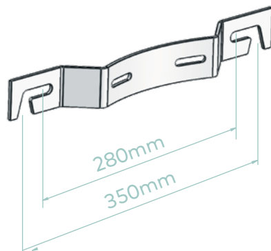
NOSAČ ZA DIRECT W modele do 150 l (fi 454mm)
