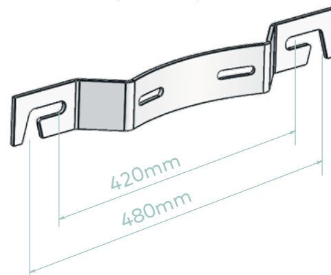
NOSAČ ZA MAX 200 modele (fi 545mm)
