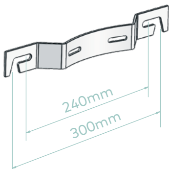
NOSAČ ZA MS modele (fi 354mm)
